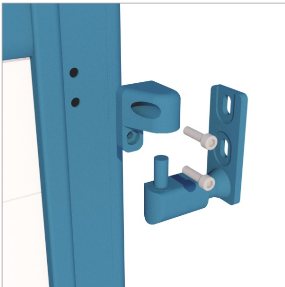
Fixation du gond
